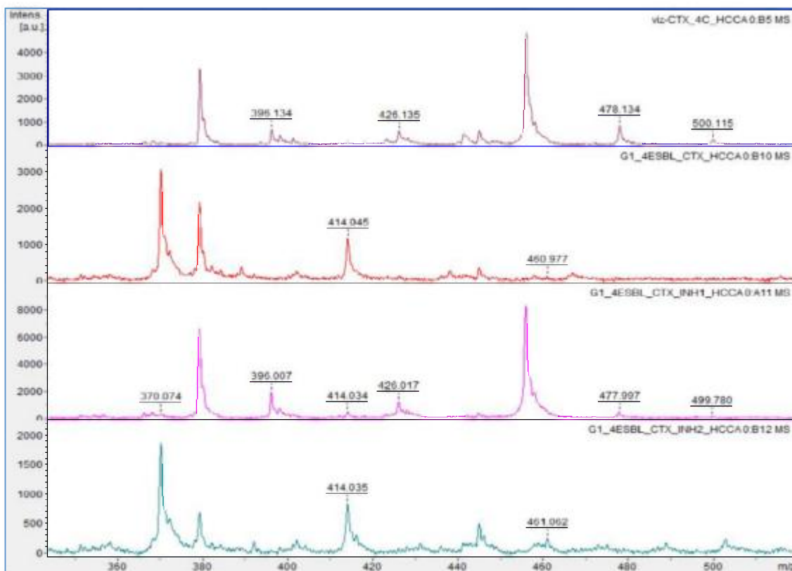
41. ábra. G1/4 E. coli + cefotaxim és inhibitorokkal végzett kísérletek spektrumai
