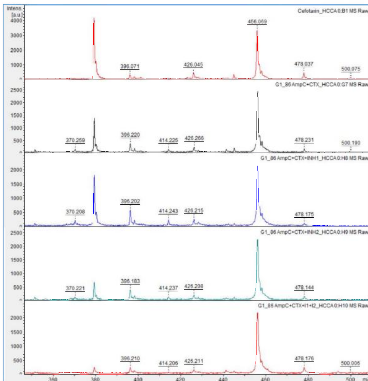
43. ábra. G1/86 Enterobacter asburiae AmpC-termelésének vizsgálata inhibitorokkal
